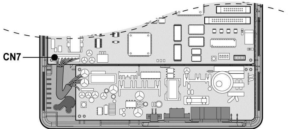
Рис. 3.2.4а Установка блока питания
