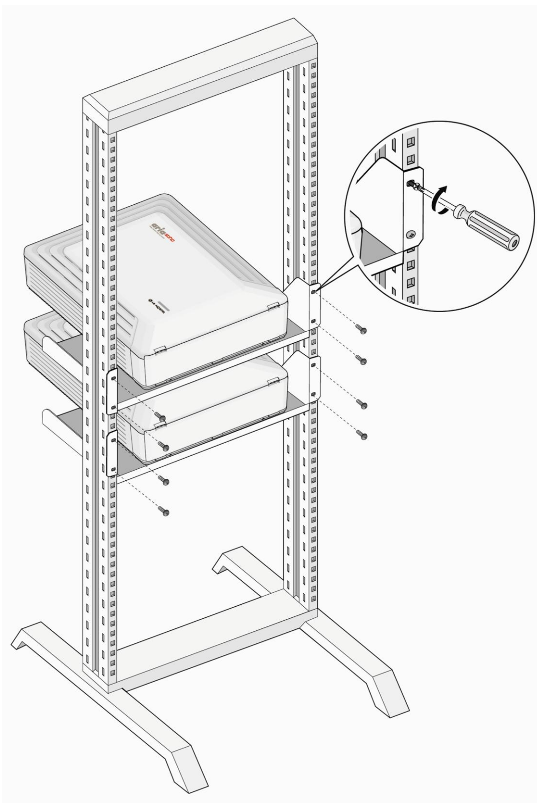
Рис. 3.3.2.26 Монтаж системного блока расширения в стойке
