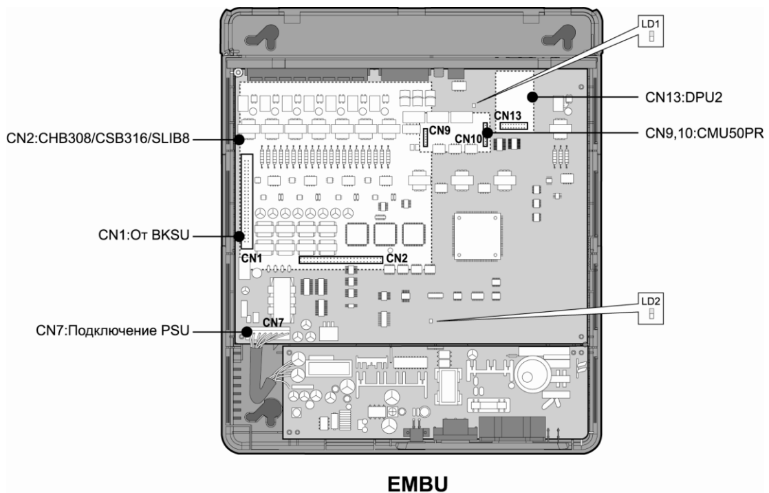
Р и с . 4.3а Материнская плата блока расширения (EMBU)
