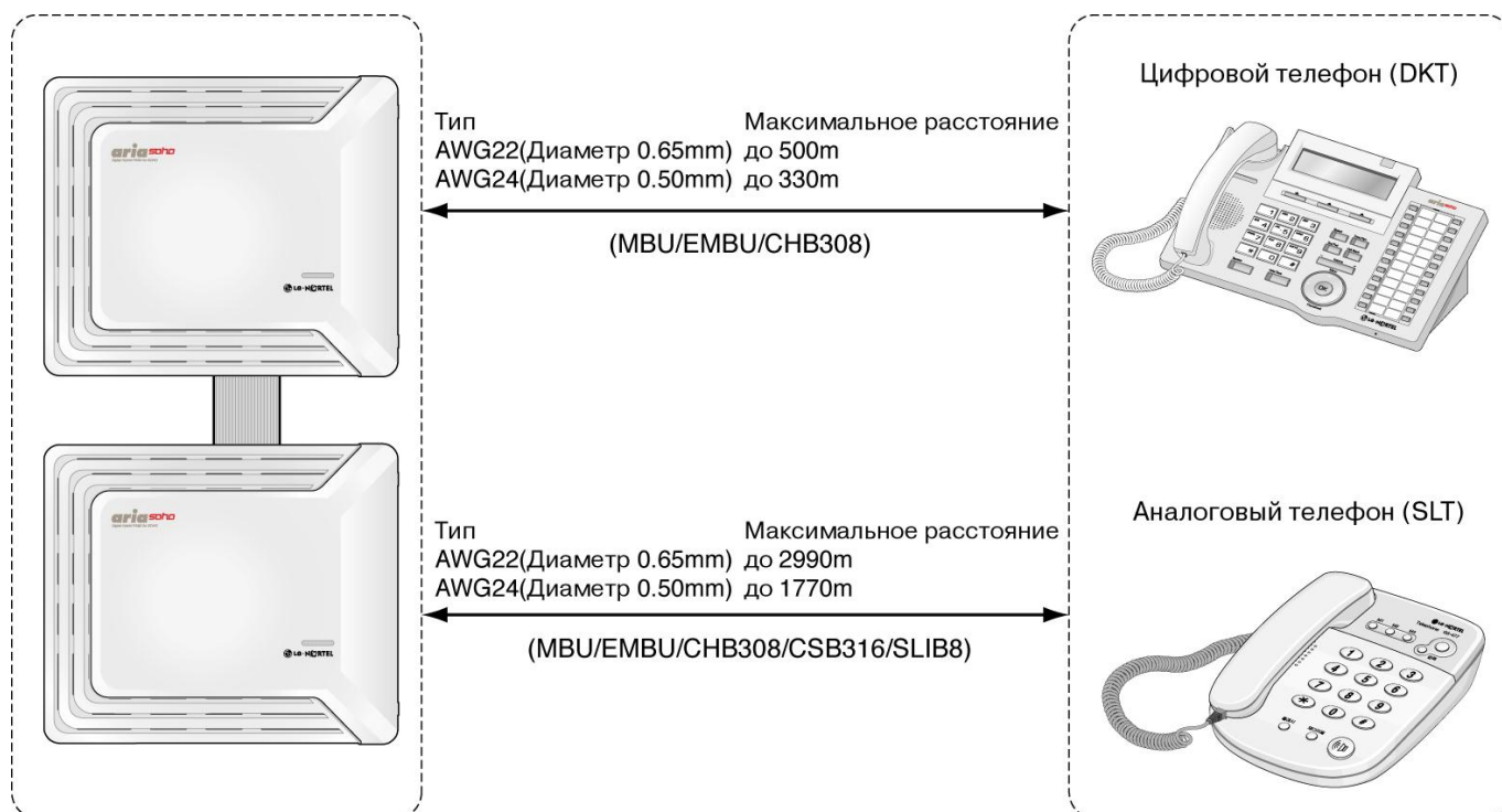
Рис. 5.1.1 Максимальная удаленность терминалов
