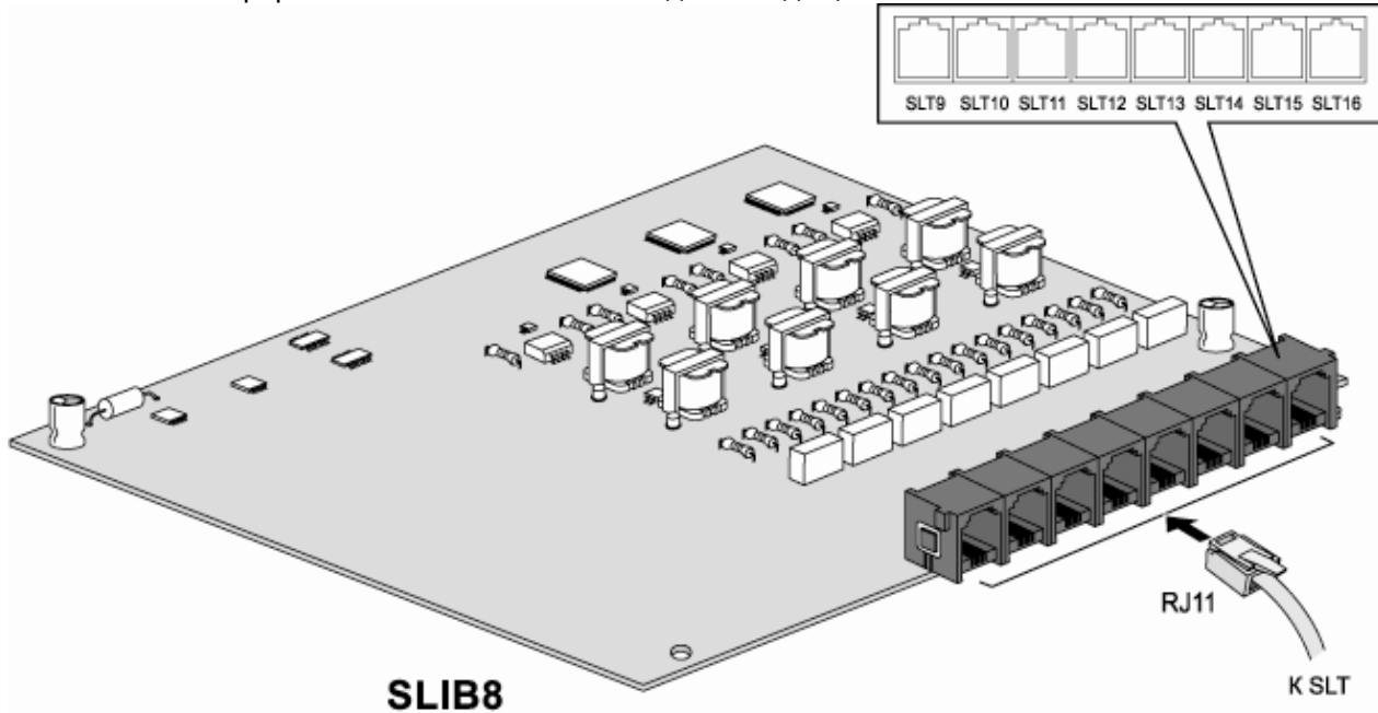
Рис. 4.4.3 Плата аналоговых абонентов SLIB8
