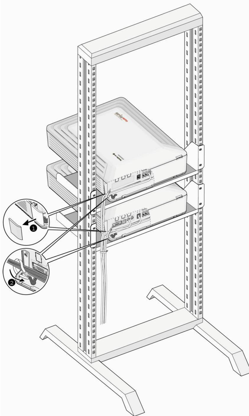
Рис. 5.2.1 Прокладка кабелей при монтаже в стойку
