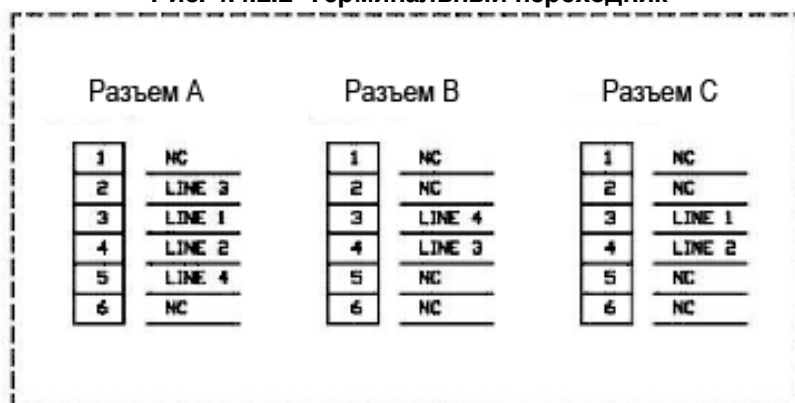
Рис. 4.4.2.2 Терминальный переходник
