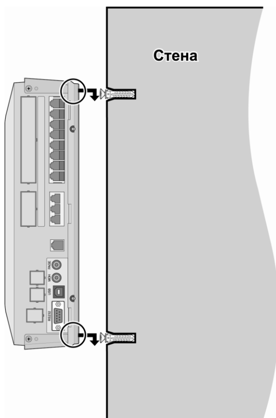
Рис. 3.2.7.16 Настенный монтаж системного блока
