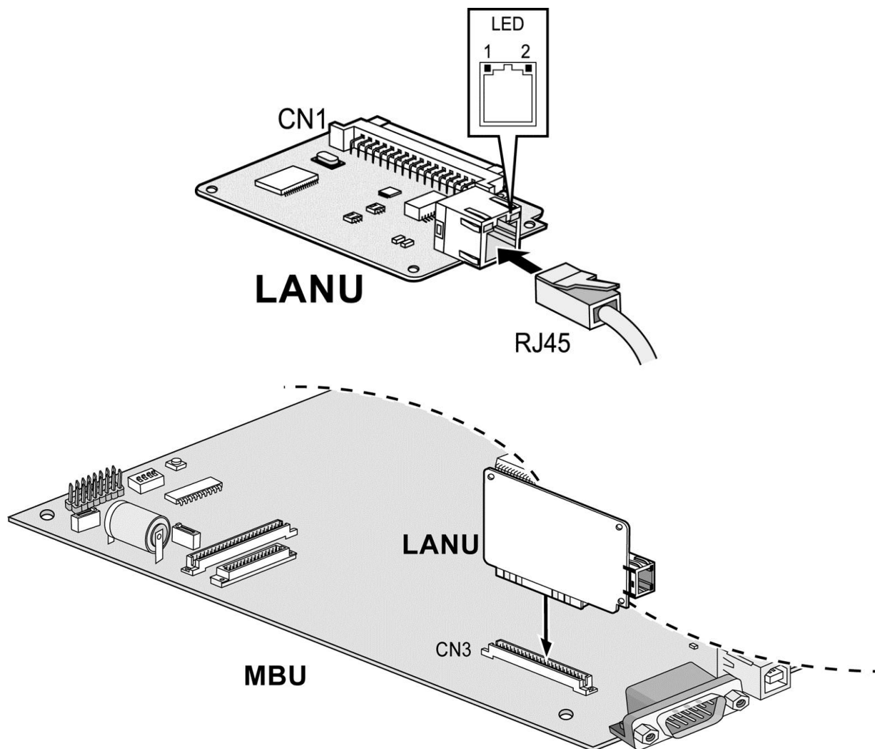
Рис. 4.5.3 Сетевой модуль LANU
