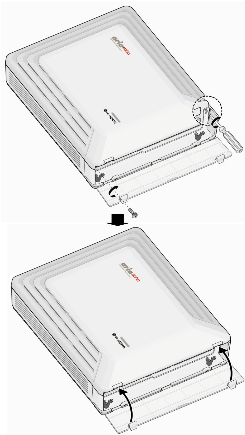
Рис. 3.2.3.2 Установка лицевой панели
