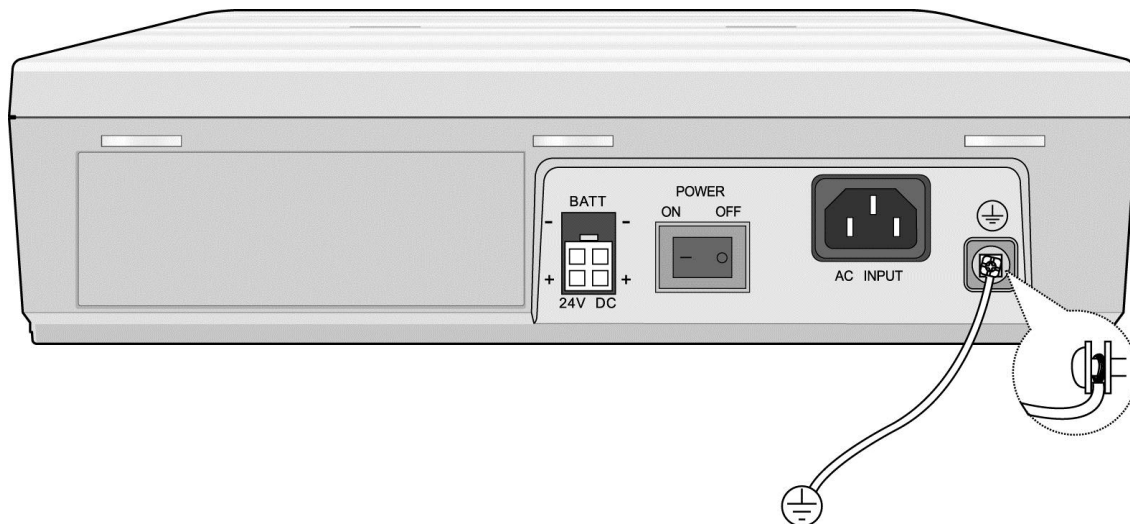
Рис. 3.2.5 Заземление корпуса
