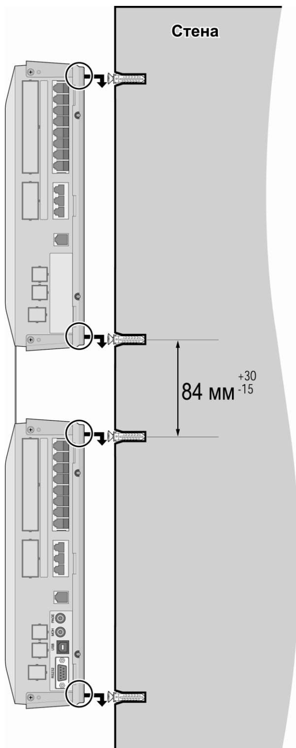
Рис. 3.3.2.16 Настенный монтаж блоков
