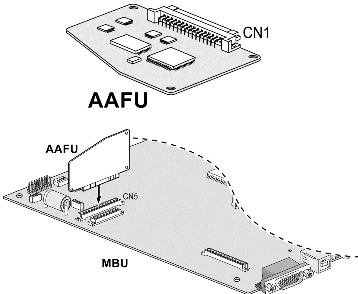
ис. 4.5.2 Плата автоматического оператора AAFU
