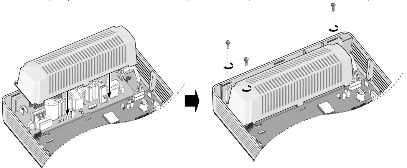
Рис. 3.2.4б Установка блока питания
