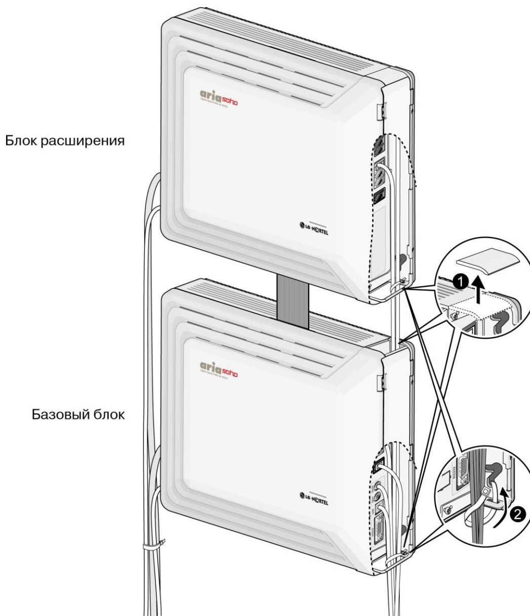
Рис. 5.2.1 Прокладка кабелей при настенном монтаже
