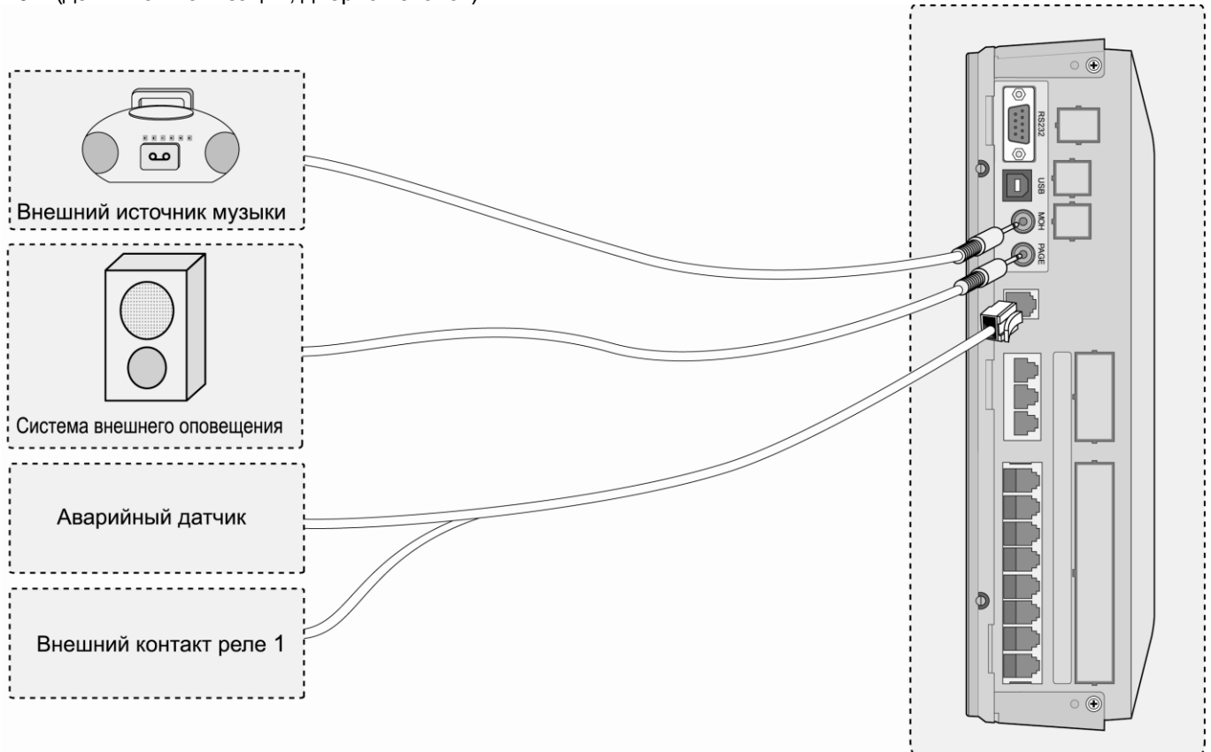
Рис. 5.1.3 Подключение дополнительных устройств
