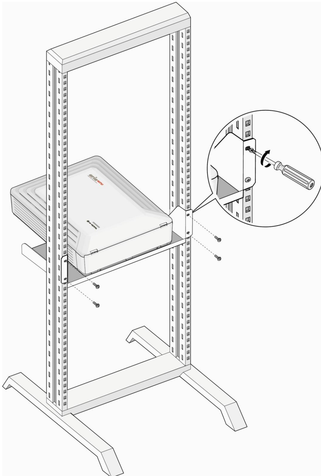
Рис. 3.2.7.2а Монтаж системного блока в стойке
