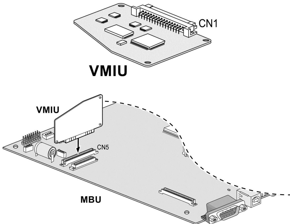
Рис. 4.5.1 Плата голосовой почты VMIU
