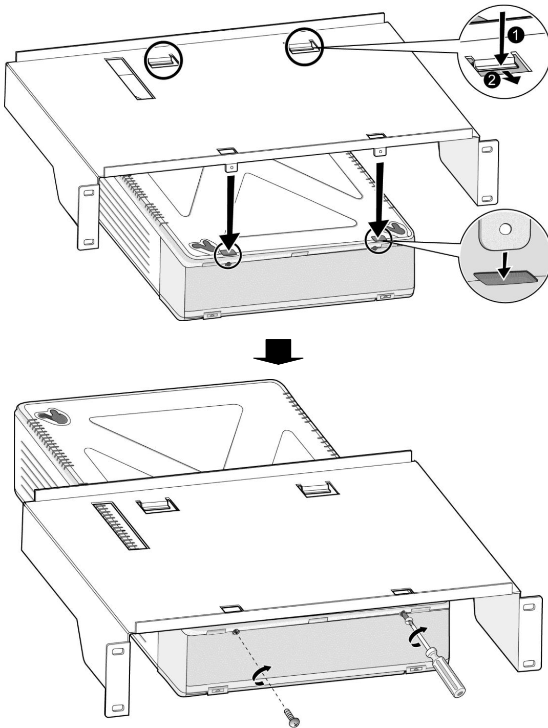
Рис. 3.3.2.a Установка стоечного крепления
