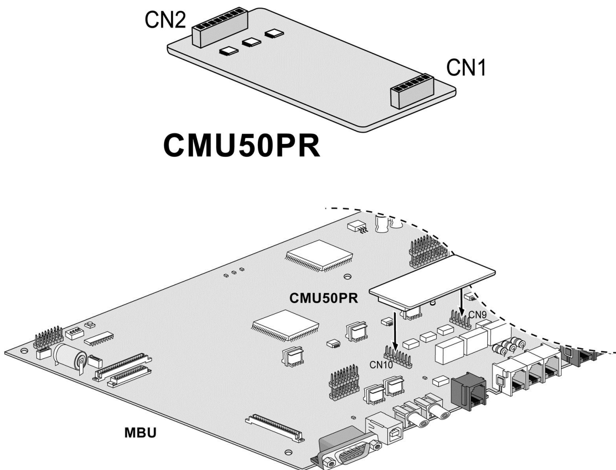
Рис. 4.5.6 Модуль определения импульсов тарификации CMU50PR
