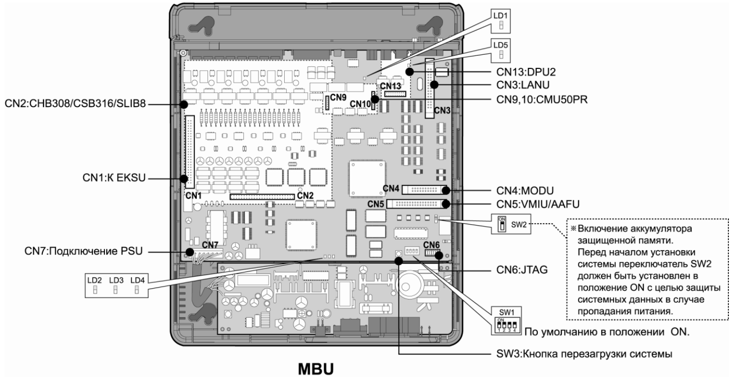
Р и с . 4.2а Материнская плата базового блока (MBU)
