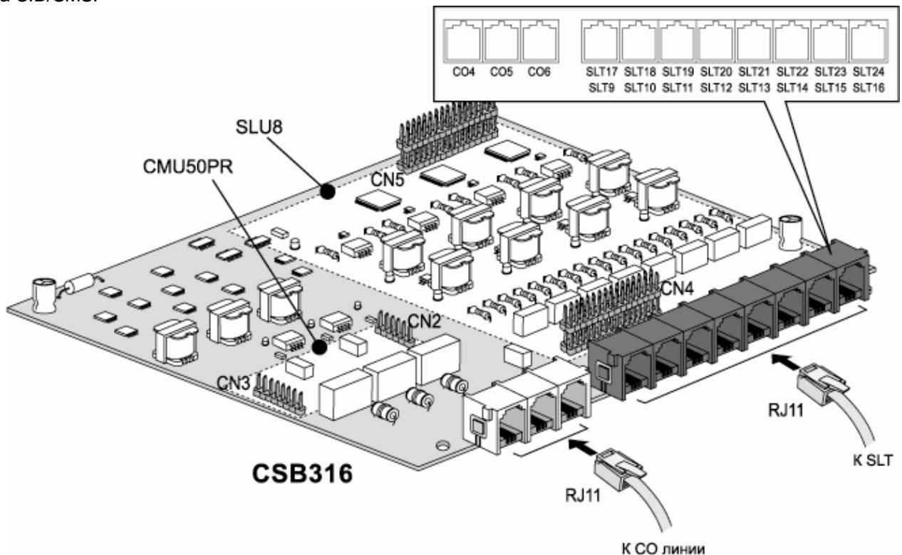
Рис. 4.4.2.1 Плата 3-х внешних линий и 16-и аналоговых абонентов (CSB316)
